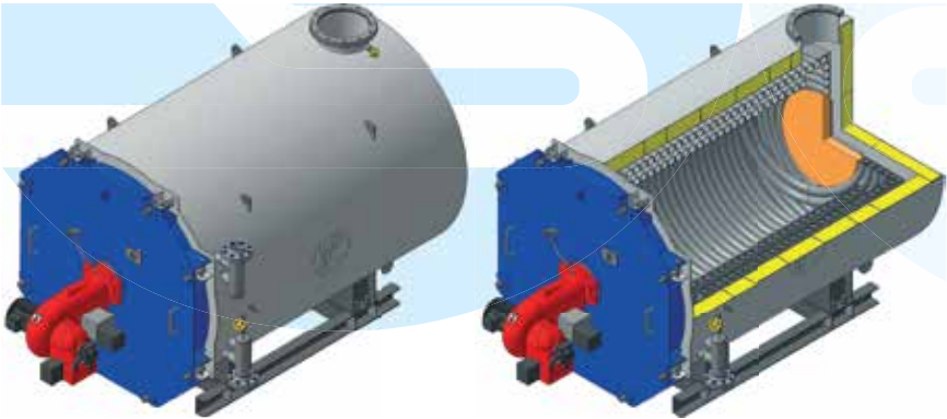
Горизонтальное исполнение
